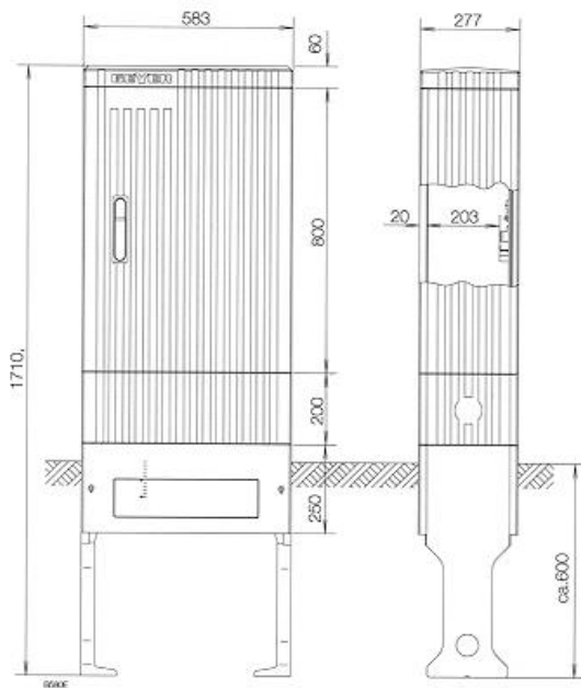
KÖRVONALRAJZ:
