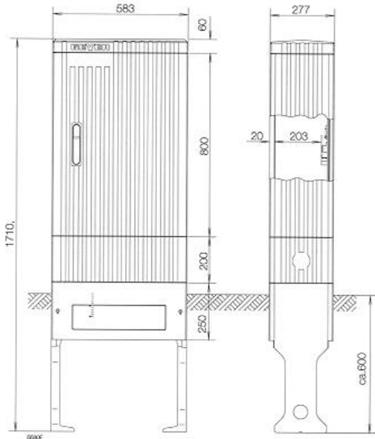
KÖRVONALRAJZ:
