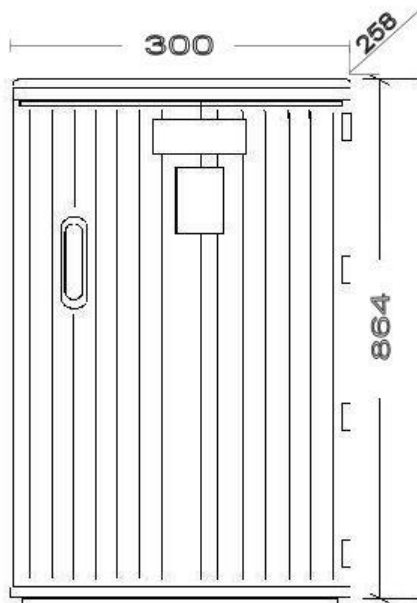
KÖRVONALRAJZ:
